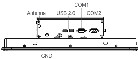
Left I/O
