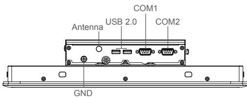
Left I/O
