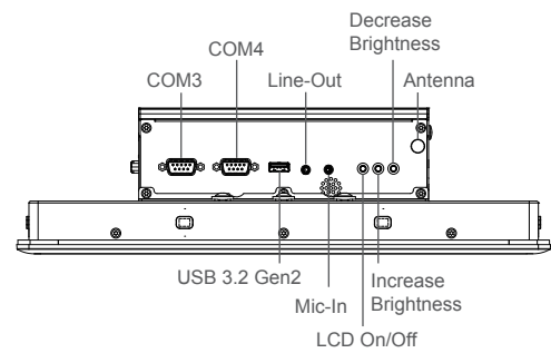
Right I/O
