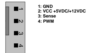
Fan - X51
