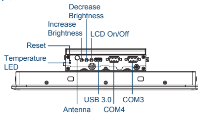
Left I/O
