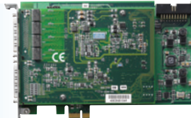
DAQe-2200
